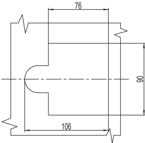
开孔尺寸 Panel Cutout
