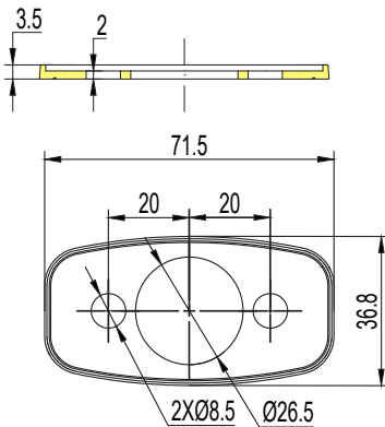
开孔尺寸Cut out
